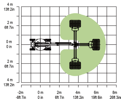
Curva de amplitud de plataforma ZA10RJE
